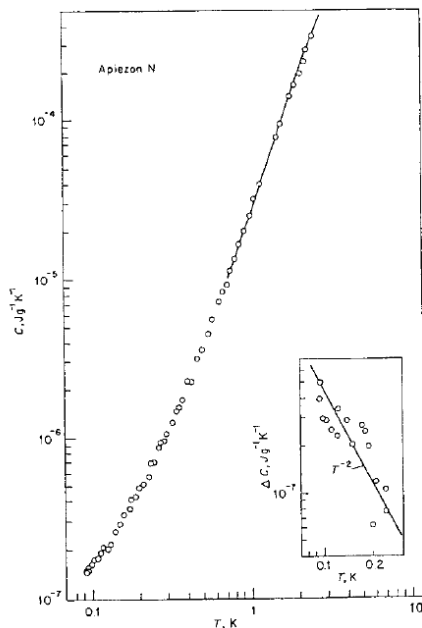
Рис. 1 Удельная теплота C смазки Apiezon N в зависимости от температуры T на графике в двойном логарифмическом масштабе. Сплошная линия представляет данные измерений Вуна и Филиппса. 4 На вставке показан частный привзнос \Delta C в зависимости от T , рассчитанный по большой постоянной времени на графике в двойном логарифмическом масштабе (см. текст)
